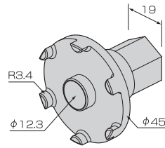
■寸法図
