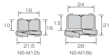
■寸法図
