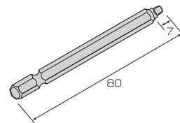
■寸法図
