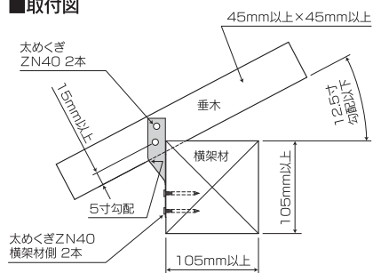
■取付図
