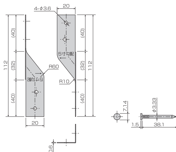
■寸法図
