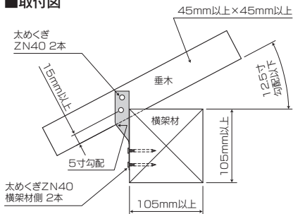
■取付図
