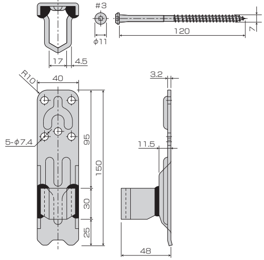
■取付図
