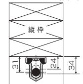
M16ボルトの設置範囲
