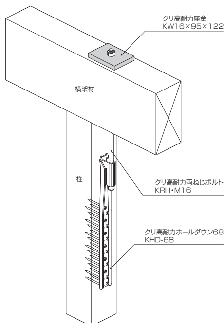
■取付図
