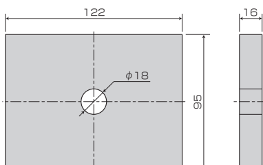
■寸法図
